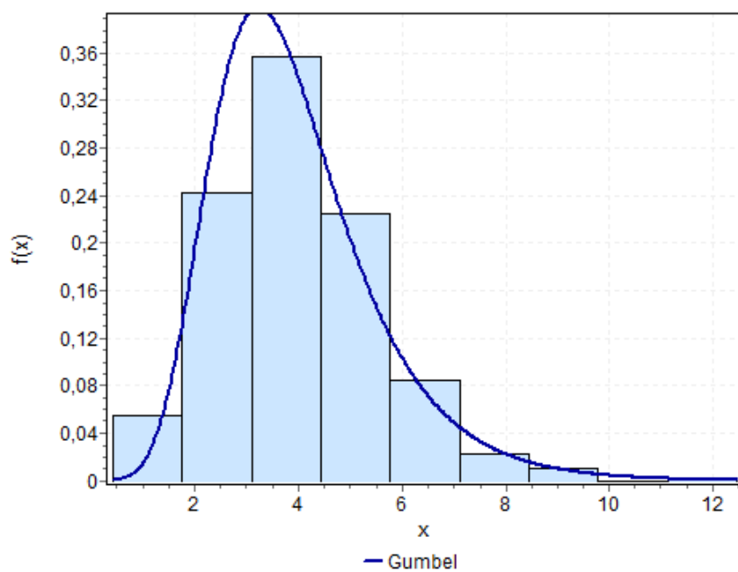
Figura I.10 – Histograma e função de distribuição de probabilidades da variável ação acidental para biblioteca.
