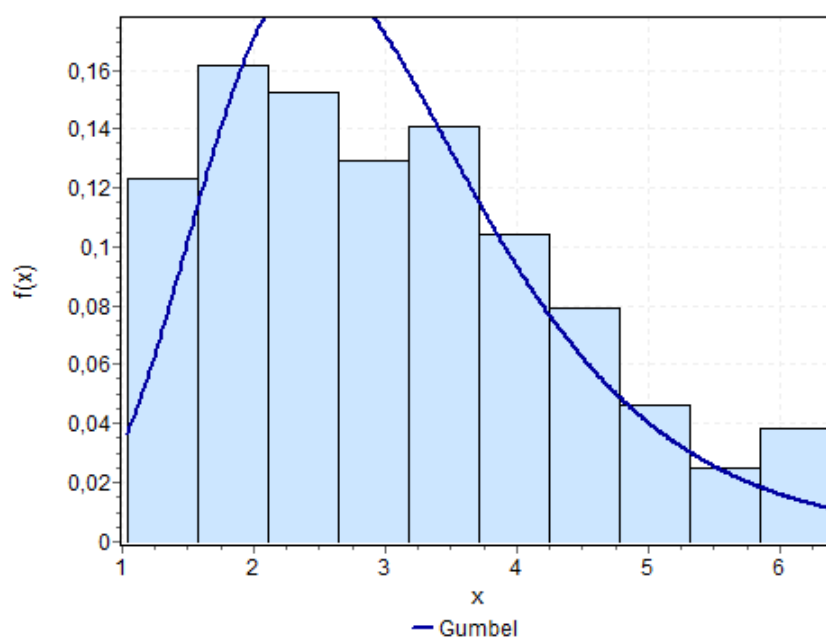
Figura I.9 – Histograma e função de distribuição de probabilidades da variável ação acidental para escola.
