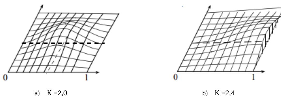
Figura 3.2 – Fator de forma da ação variável do tipo acidental (Adaptado do JCSS, 2001).
