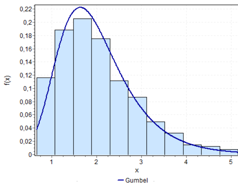
Figura I.8 – Histograma e função de distribuição de probabilidades da variável ação acidental para hospital.
