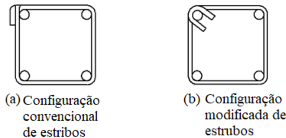
Figura 12. Configuração da armadura da seção transversal convencional (estribos) de um pilar de concreto de alta resistência (a) e configuração modificada para melhor (b) (Kodur et al., 2005).
