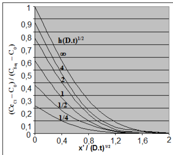
Figura 4: Curvas de relação entre (C_{Cl} - C_0) / C_{Seq} - C_0 e (x' / 2(D.t)^{1/2}) [5]
