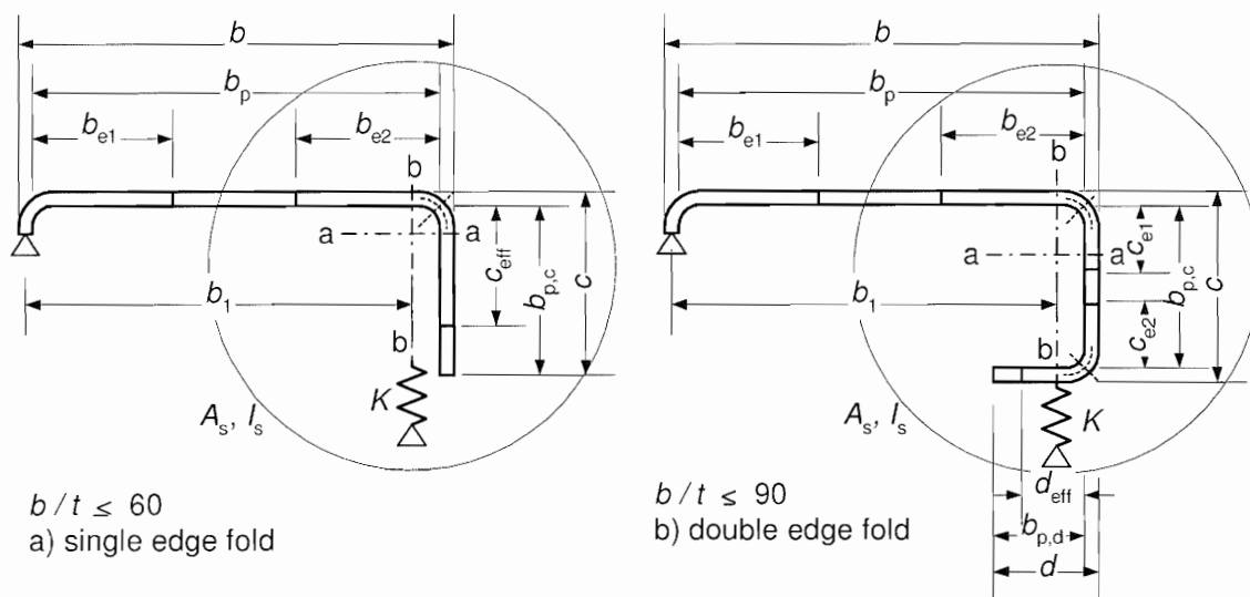
Figure 5.7: Edge stiffeners
