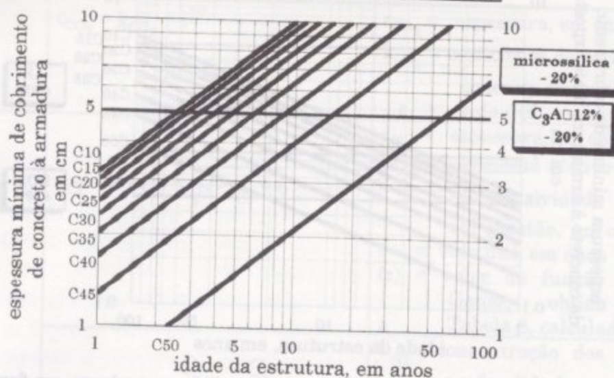
Figura 7. Ábaco para obtenção da espessura de cobrimento às armaduras em função do ambiente (zona urbana, industrial, marinha ou rural), do concreto (C10 a C50) e da vida útil desejada (1 a 100 anos). Caso sejam utilizadas adições de 8% de sílica ativa ou empregados cimentos Portland com teor de C_3A \leq 12\% , as espessuras mínimas características de cobrimento de concreto à armadura, podem ser reduzidas em 20%. Ábacos similares são disponíveis para outras condições de exposição.
